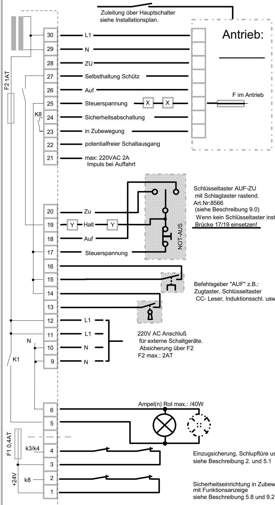
Steuerplatine TST 90/1
